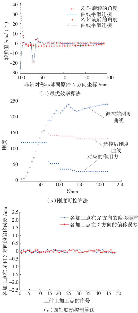
图9 开发的几种气囊抛光控制算法
