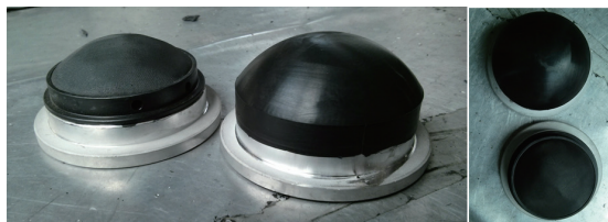
图7 设计的柔性气囊及其结构 Fig.7 Bonnet polishing head
