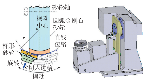
图3 2轴杯形砂轮修整装置
