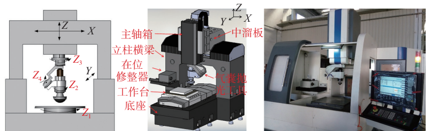
图6 可控气囊抛光样机模型和实物图
