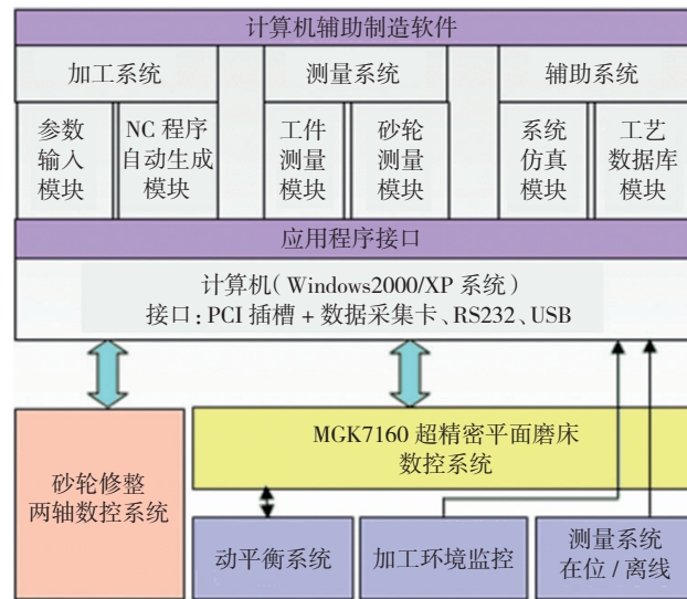
图4 大口径非球面精密磨削加工计算机辅助制造软件
